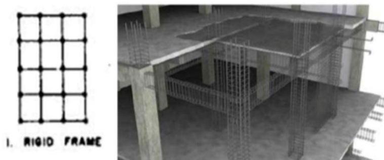
Gambar 12. Sistem Rangka Kaku (kolom dan balok)
