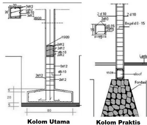
Gambar 11. Pondasi
