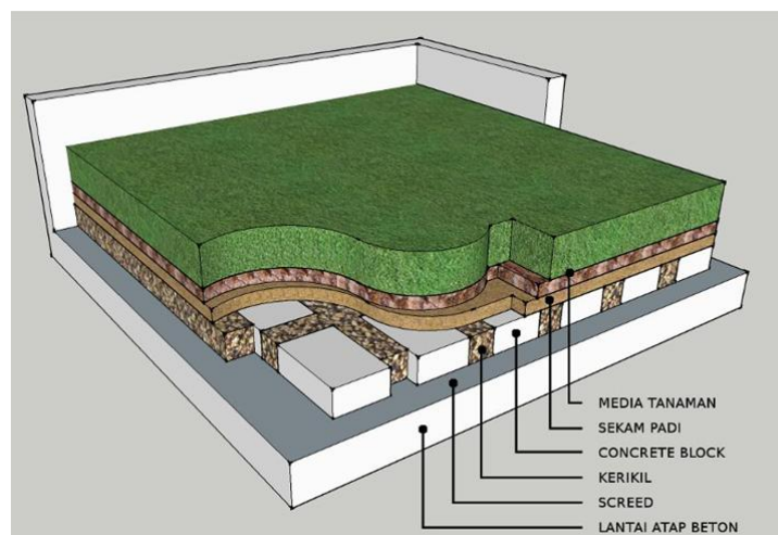
Gambar 13. Struktur Green Roof
